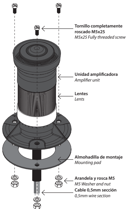
Montaje boca abajo. Upside down mounting.
